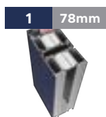
1 78mm Ciepła ościeżnica z poliamidową przekładką termo- izacyjną
