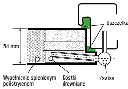
PROFIL SKRZYDŁA
