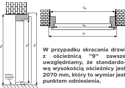
Wymiarowanie drzwi z ościeżnicą „9”
