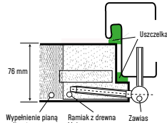
PROFIL SKRZYDŁA
