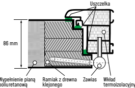
PROFIL SKRZYDŁA
