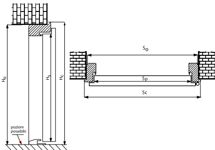
Wymiarowanie drzwi z ościeżnicą ALU HYBRID
