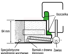
PROFIL SKRZYDŁA
